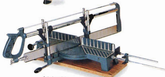
Scie à onglets
