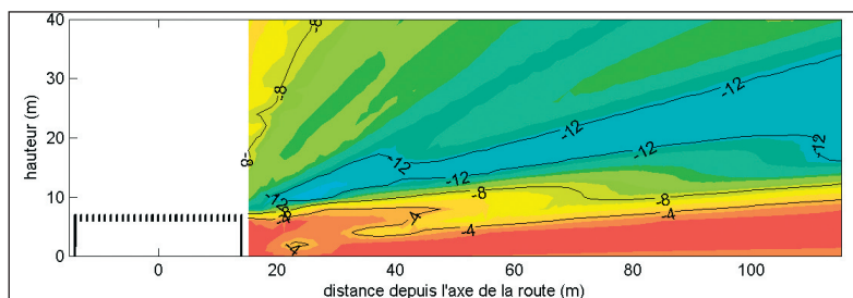
^ Efficacité acoustique d'une couverture ajourée, calcul MICADO
